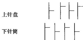
图2 提花网眼复合织物的织针排列图
