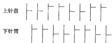
图1 针织网眼织物织针排列图
